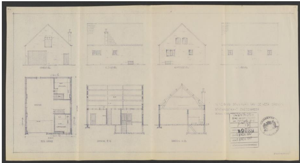
Tekening uit de serie gedigitaliseerde bouwdoSSIers uit de periode 1940-1950
